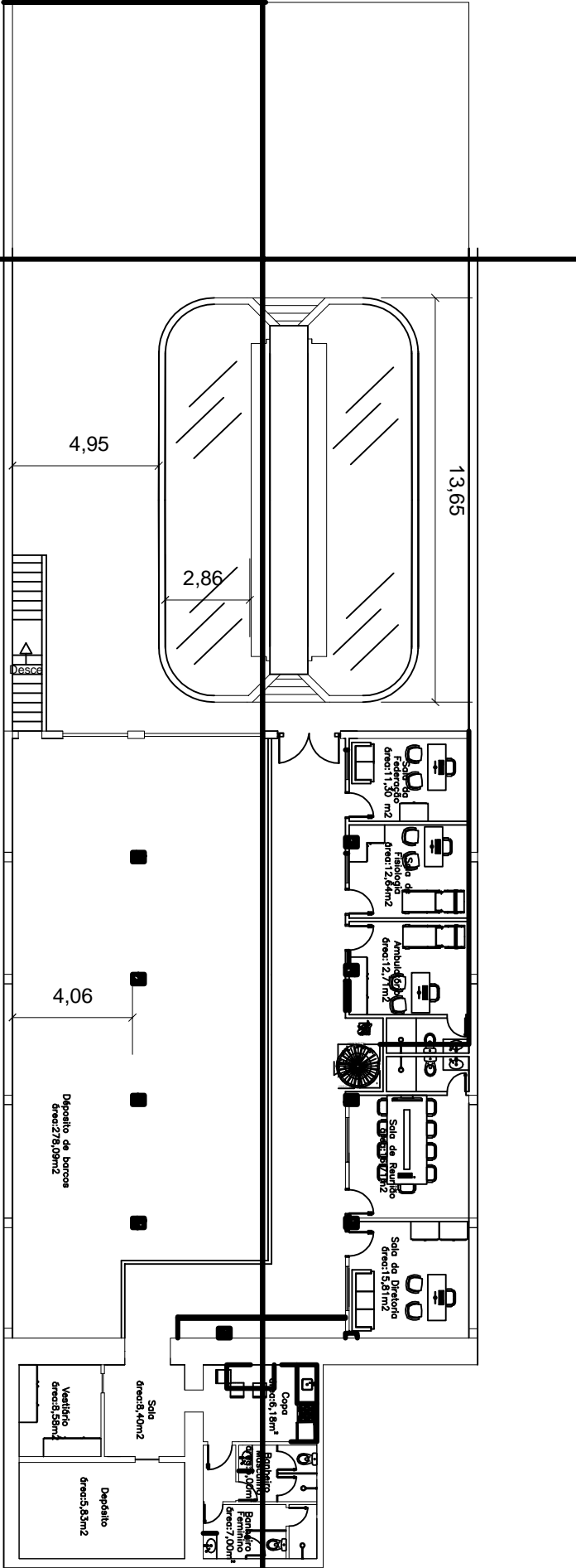
Planta Baixa - Nível Inferior Sede do Paysandu
